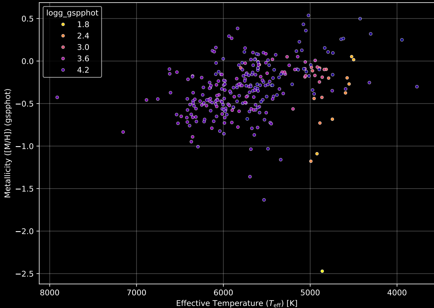
GALAH DR4 Field: [1240] Stellar Population Parameters (n= 282)
