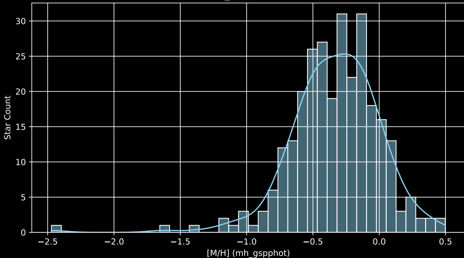
GALAH DR4 Field: [1240] [M/H] (mh_gspphot) (n= 281)
