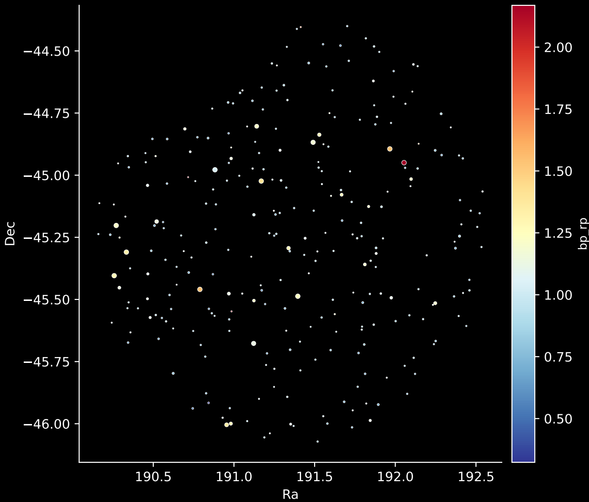
GALAH DR4 Field: [1240] Stars: 282
